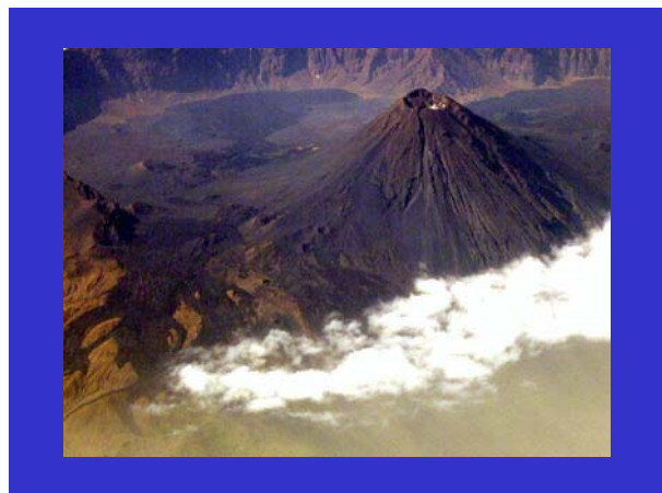
Fogo Volcano Cabo Verde
